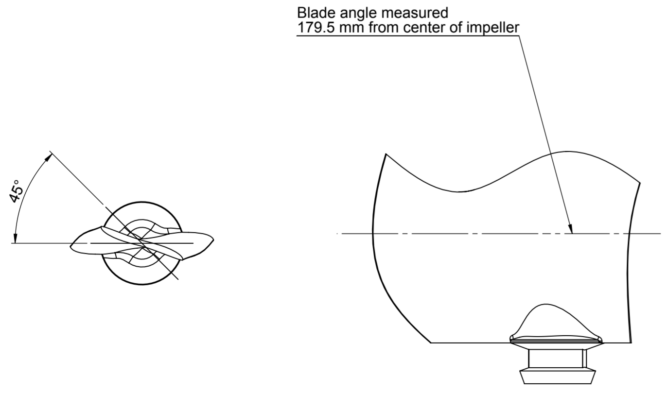
Blade Angle
